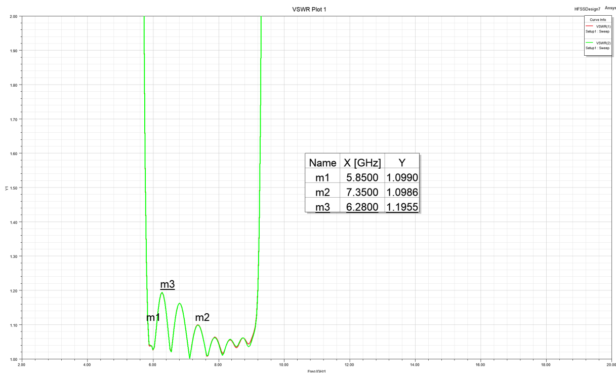
驻波-VSWR
